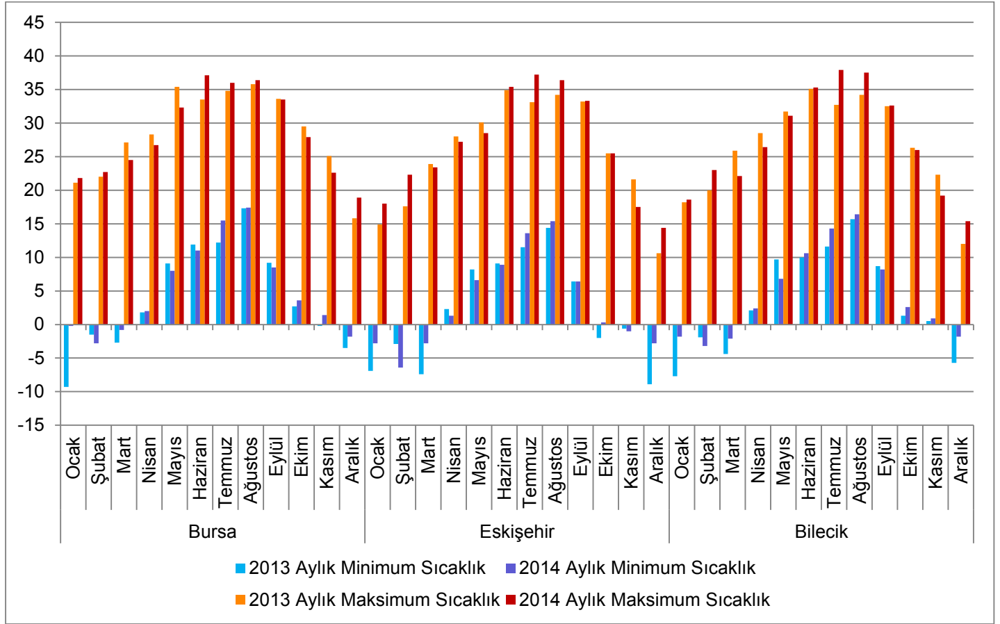
Grafik 1. 2013-2014 Yılları Aylık Minimum ve Maksimum Sıcaklıklar (°C)
