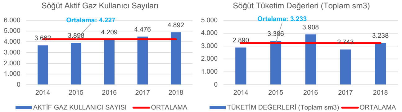
Şekil 7. Söğüt İlçesi Doğalgaz Kullanımı (2014-2018)
